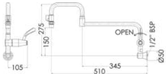
T-3MPKW
